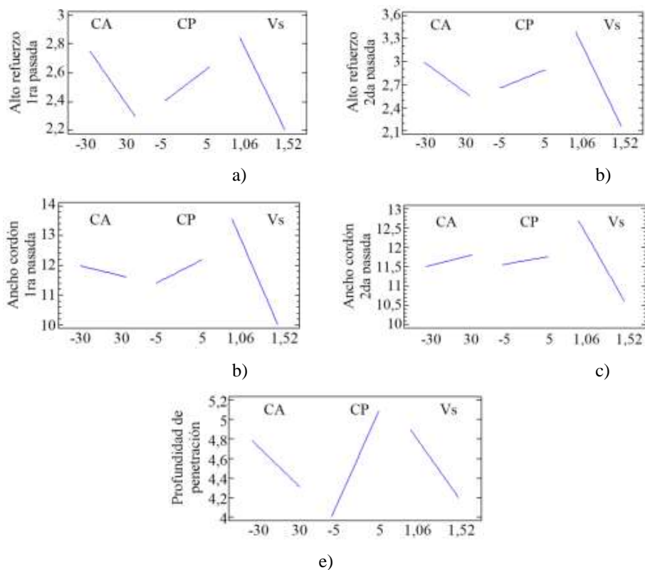
Figura 4. Gráfica de efectos principales. Elaboración propia.
