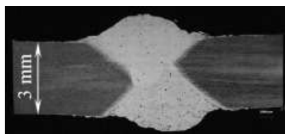
A1. CA= + 30 %; CP= + 5 %; v_s = 1,52 \text{ cm}\cdot\text{s}^{-1}
