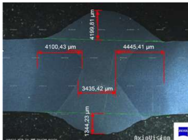
Figura 3. Ejemplo de medición de los parámetros geométricos de las uniones. Elaboración propia
