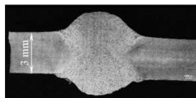
A3. CA= + 30 %; CP= - 5 %; v_s = 1,06 \text{ cm}\cdot\text{s}^{-1}
