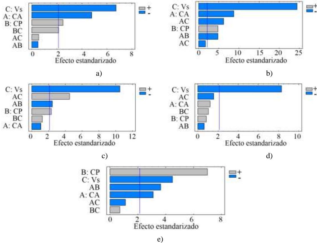
Figura 5. Diagrama de Pareto estandarizado. Elaboración propia
