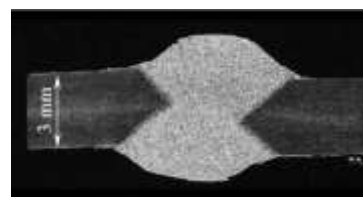
A7. CA= - 30 %; CP= - 5 %; v_s = 1,06 \text{ cm}\cdot\text{s}^{-1}
