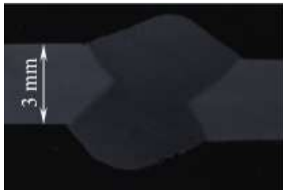
A9. CA= + 30 %; CP= + 5 %; v_s = 1,52 \text{ cm}\cdot\text{s}^{-1}
