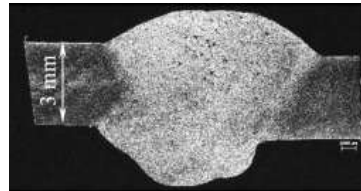
A11. CA= + 30 %; CP= - 5 %; v_s = 1,06 \text{ cm}\cdot\text{s}^{-1}
