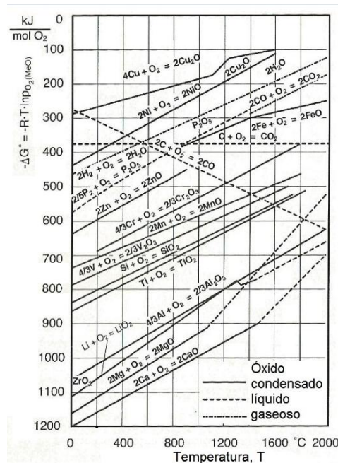
Figura 1. Diagrama de Ellingham (Chalmers, 1968)
