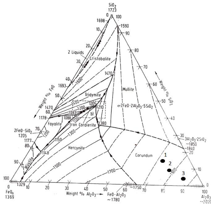
Figura 3. Diagrama de fase \text{Al}_2\text{O}_3\text{-FeO-SiO}_2 (Slag atlas, 1981)
